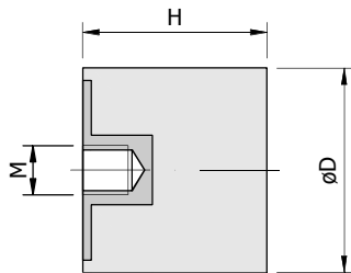
Odbojnik gumeni Tip-B ØD x H ; M
