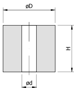
Spojnički uložak gumeni Tip-B \varnothing D / \varnothing d \times H
