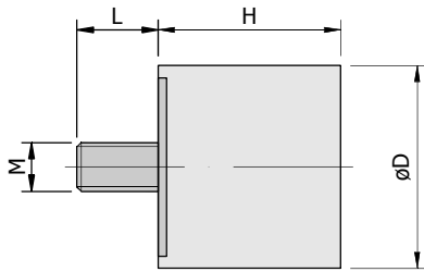
Odbojnik gumeni Tip-A ØD x H ; M x L
