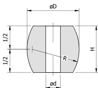
Spojnički uložak gumeni Tip-D \varnothing D / \varnothing d \times H ; R
