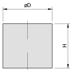
Spojnički uložak gumeni Tip-A \varnothing D \times H
