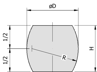
Spojnički uložak gumeni Tip-C \varnothing D \times H ; R
